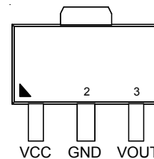
SOT-89-3
